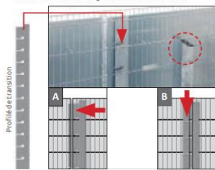
Jonction insonorisée de gabions anti-bruit attenants
